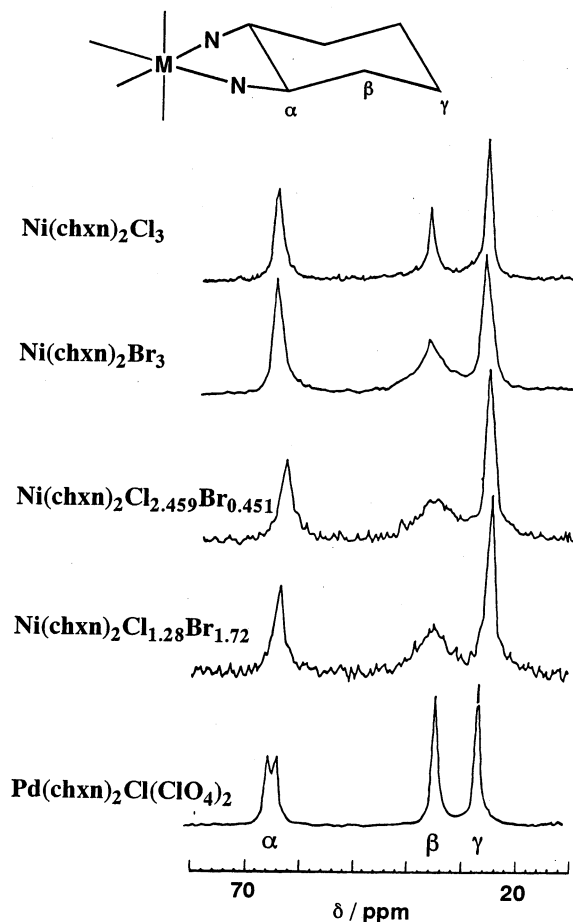
Fig. 6. CP-MAS ^{13}\text{C} -NMR spectra of \text{Ni}(\text{chxn})_2\text{X}_2 and \text{Pd}(\text{chxn})_2\text{Cl}(\text{ClO}_4)_2 .
